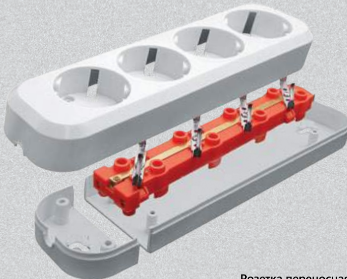
Розетка переносная STEKKER PST16-410-20 на 4 гнезда, с заземлением.
