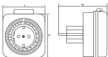
Суточный механический
